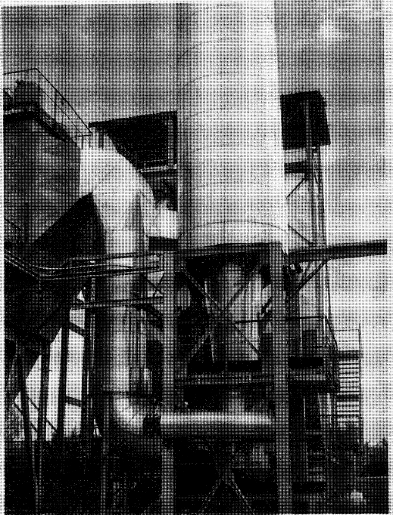
Reattore linea 2
