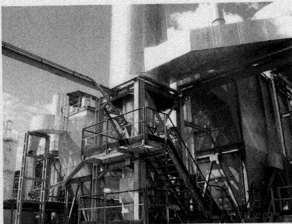
Reattore linea 1
