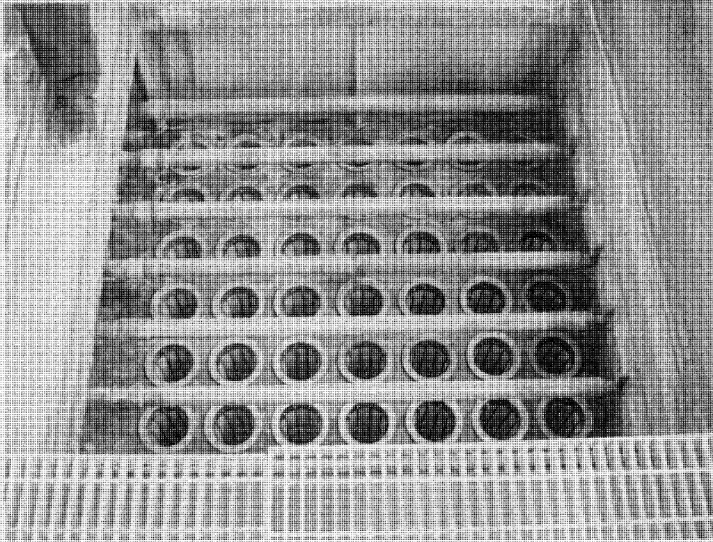
Testata filtro a maniche linea 2
