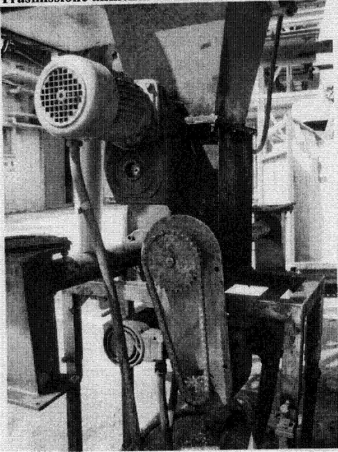
Trasmissione alimentatore carbone
